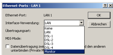
WEBconfig: LCOS-Menübaum / Setup / Schnittstellen / Ethernet-Ports
