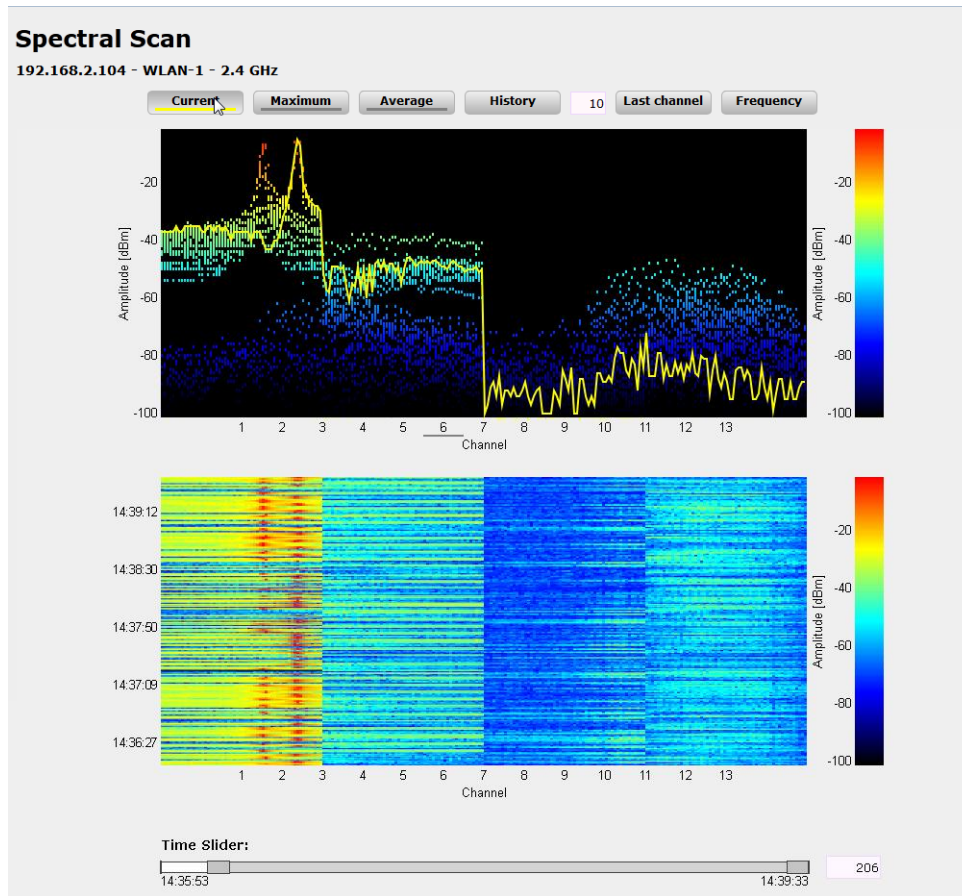
Abbildung 4: Spectral Scan, Kanal-Anzeige Current, letzte 10 History-Werte und "Time Slider", Störung durch Baby-Phone
