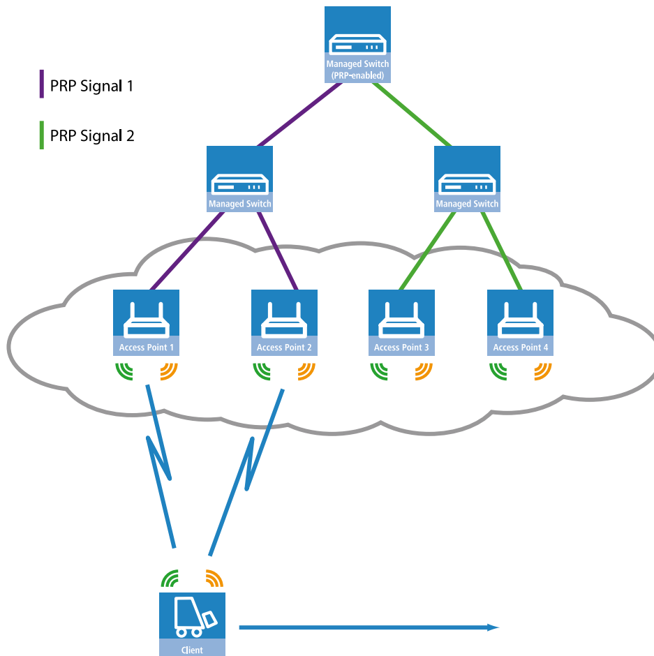
Abbildung 5: Roaming eines Dual-Radio-Clients in einer PRP-gestützten WLAN-Infrastruktur
