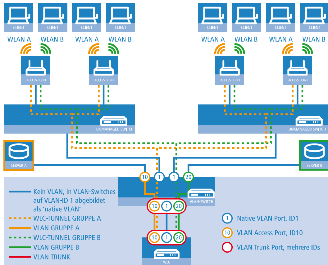
Abbildung 7: Anwendungsbeispiel Overlay-Netz
