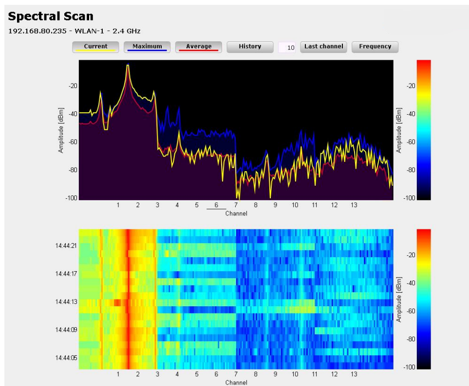
Abbildung 3: Spectral Scan, Kanal-Anzeige Current, Maximum, Average, Störung durch Funk-Kamera
