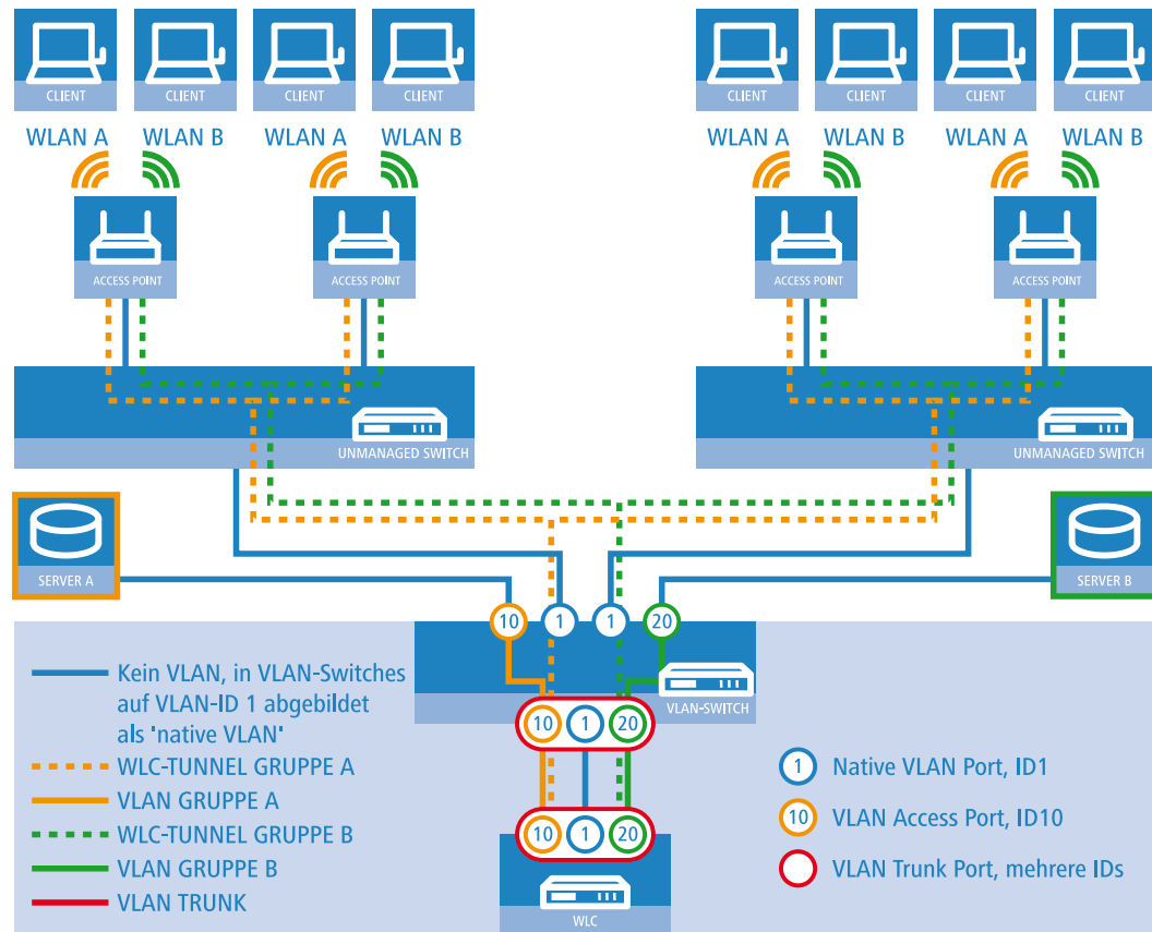
Abbildung 19: Anwendungsbeispiel Overlay-Netz
