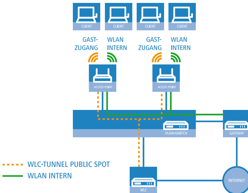
Abbildung 9: Anwendungsbeispiel WLAN-Controller mit Public Spot
