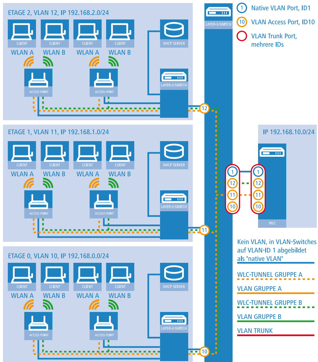
Abbildung 8: Anwendungsbeispiel Layer-3-Roaming
