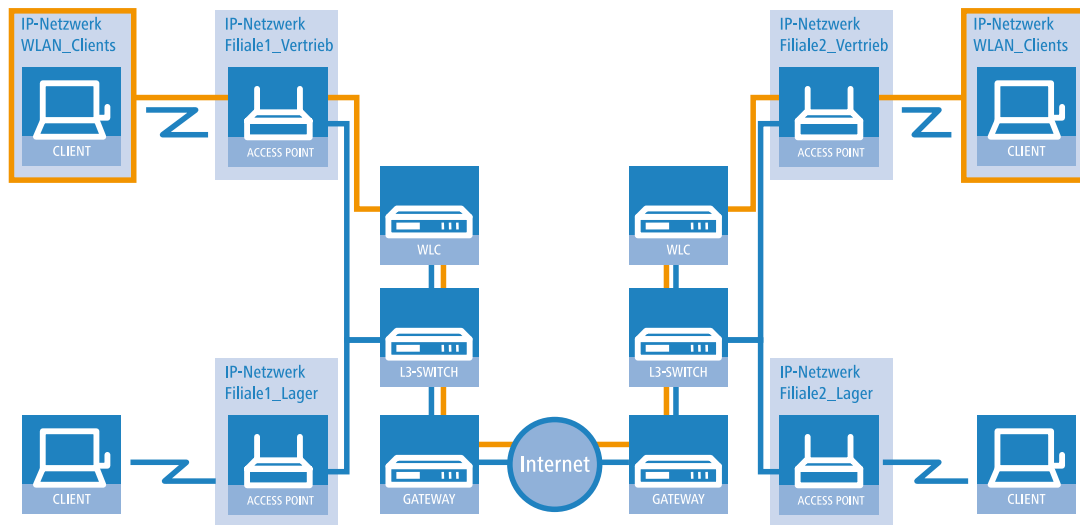
Abbildung 6: Overlay-Netzwerk über mehrere IP-Netzwerke hinweg
