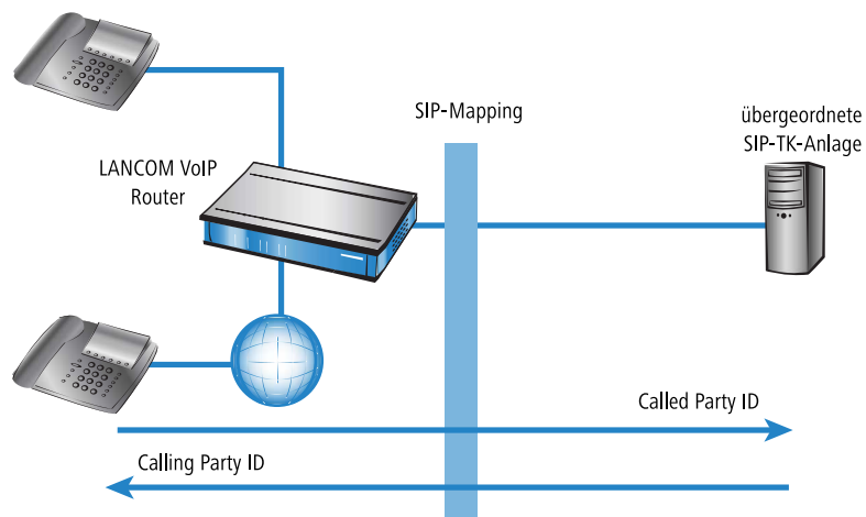
LANconfig: VoIP-Call-Manager / Leitungen / SIP-Mapping
