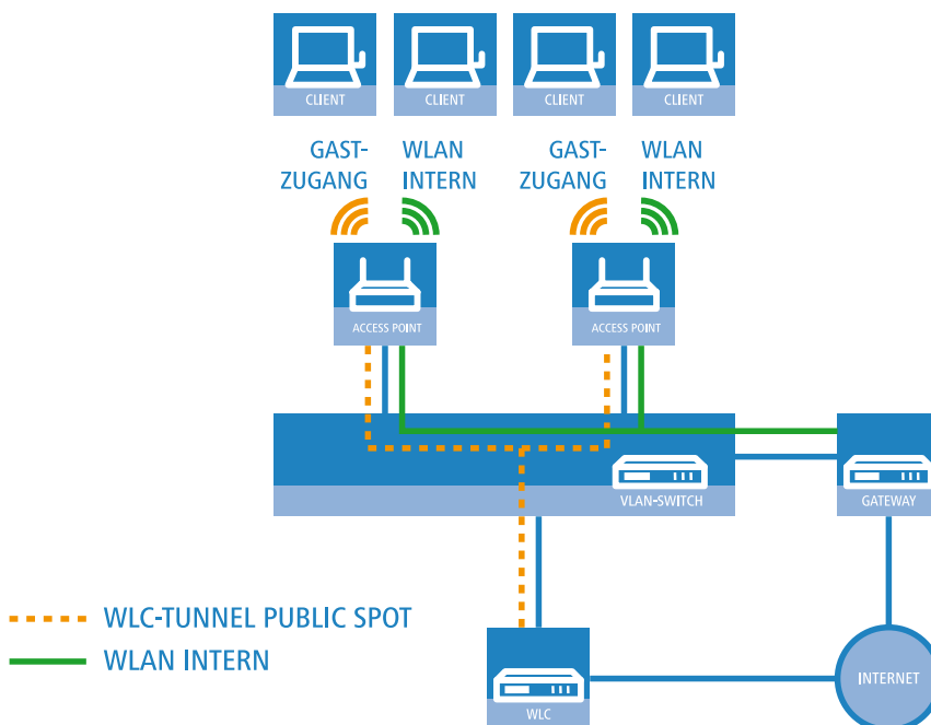
Abbildung 20: Anwendungsbeispiel WLAN-Controller mit Public Spot
