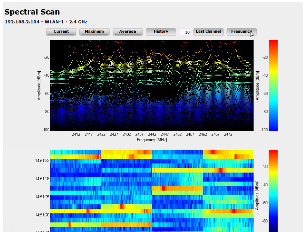
Abbildung 2: Spectral Scan, Frequenz-Anzeige der letzten 10 History-Werte
