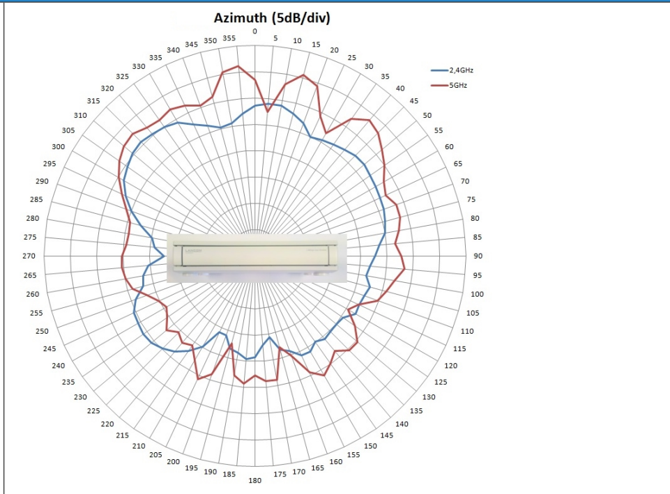
Abstrahlungsdiagramme Antennen, Frontansicht
